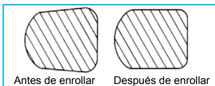
La sección transversal trapezoidal modificada de los resortes de alambre rectangular cambia a una sección transversal en "D" durante el enrollamiento para lograr un bajo nivel de esfuerzo que se traduce en una mayor vida útil del resorte.
