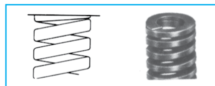
Los extremos de cada resorte están cerrados y maquinados a escuadra para asegurar que el resorte se apoye en cualquiera de sus extremos y proporcione una máxima superficie de apoyo.
